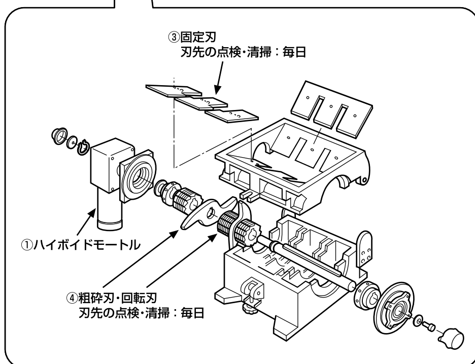
分解図
